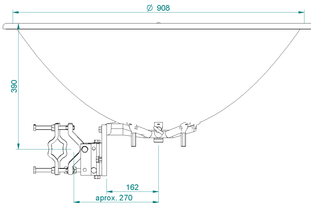
Obr. 1 Rozměry antény
