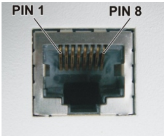
Fig. 3.7: RJ-45F
