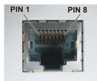
Fig. 3.4: RJ-45F
